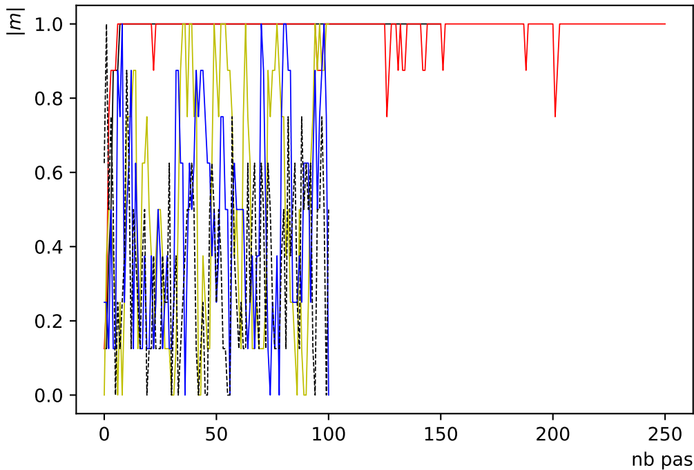
Evolution de l'aimantation sur critère Estimation par intervalle, N=4
